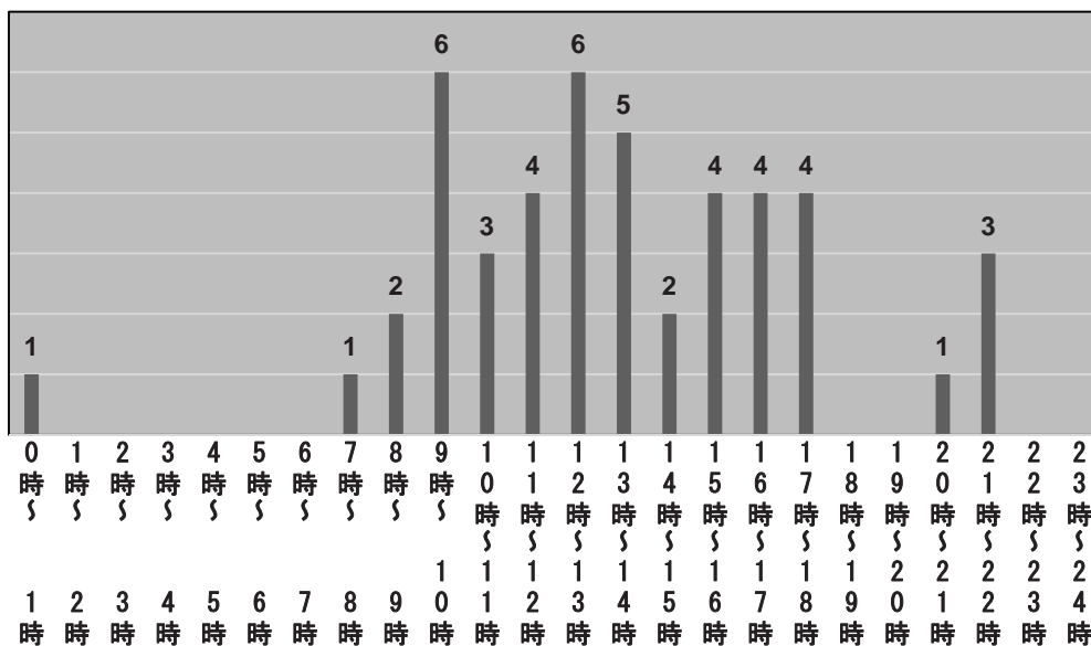
時間別件数
