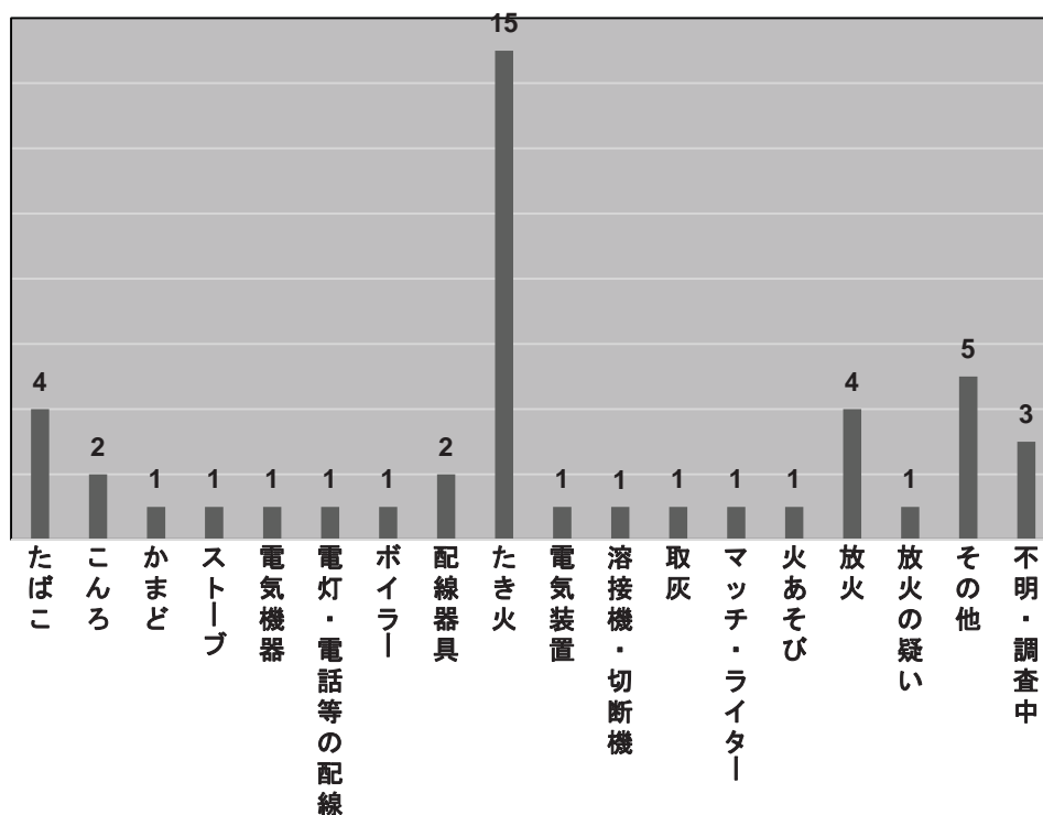
原因別件数
